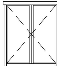
Double door 1615x1920 1pcs
